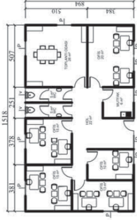
P.O.14 125 m² PREFABRİK OFİS PLANI
