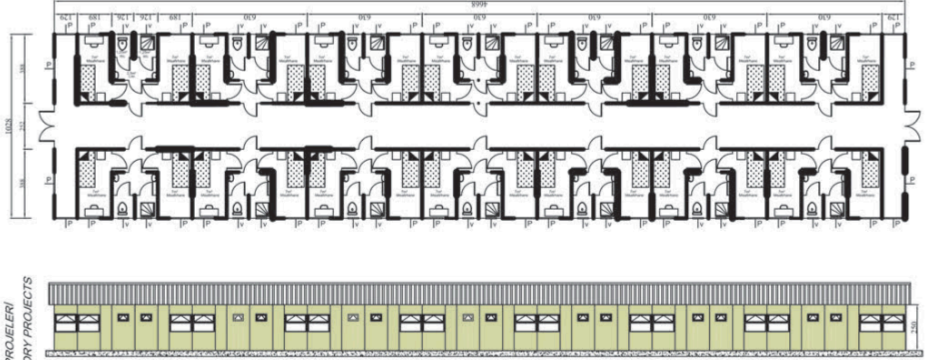
ÖN CEPHE GÖRÜNÜMÜ FRONT VIEW
