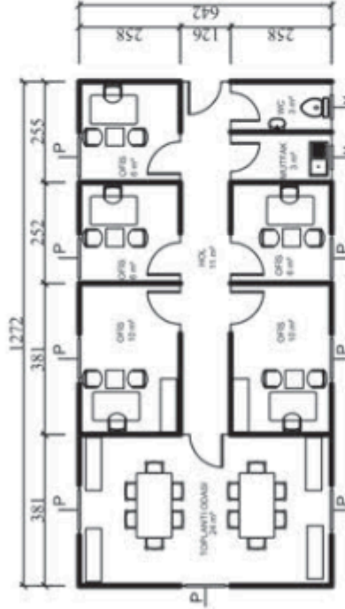
78 m² Prefabrik Ofis Planı
