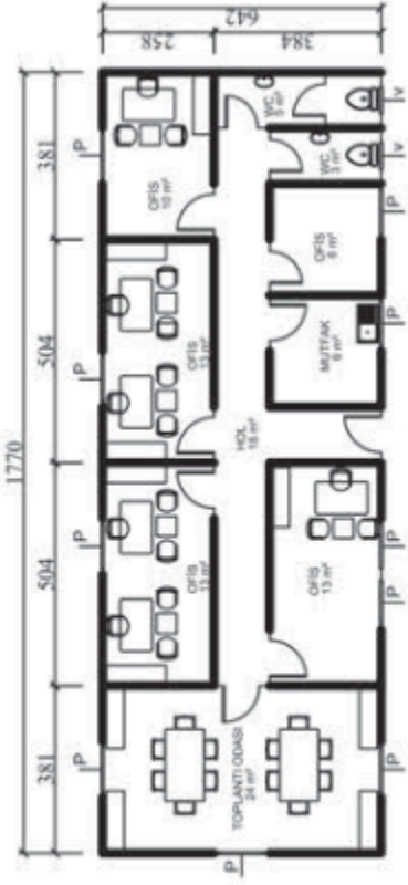
P.O.13 114 m² PREFABRİK OFİS PLANI
