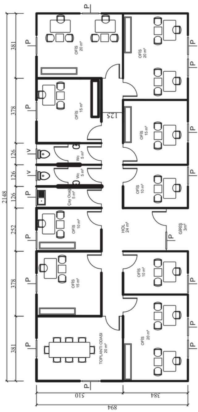
P.O.19 192 m² PREFABRİK OFİS PLANI
